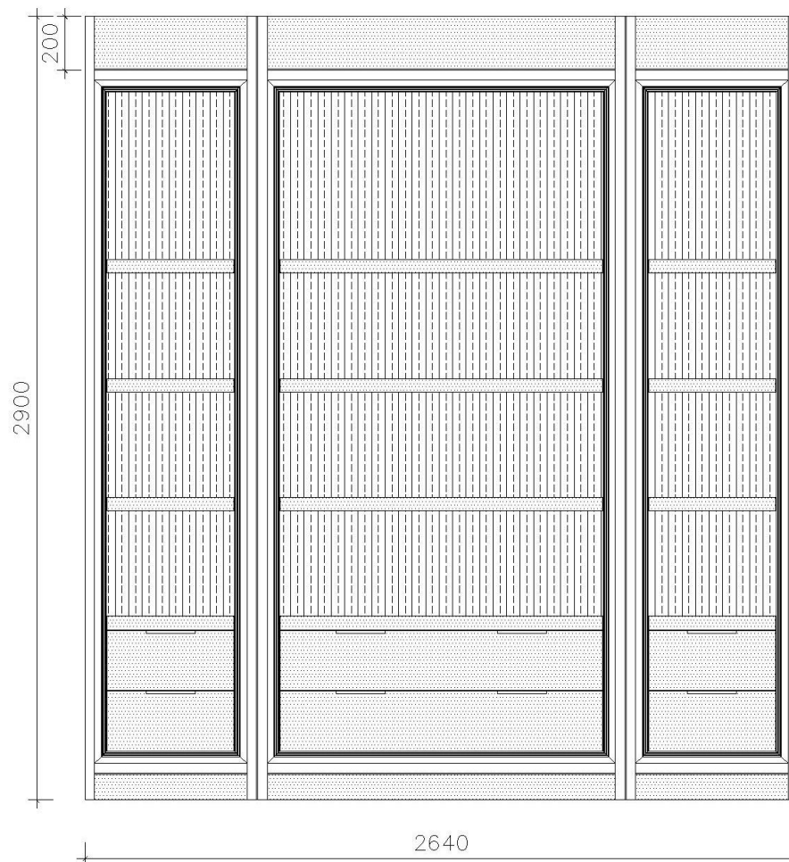
2 01 正立面图 SCALE 1/30
