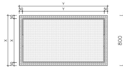
顶面图 SCALE 1/20
