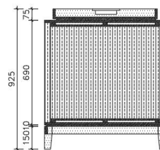
剖面图 SCALE 1/20
