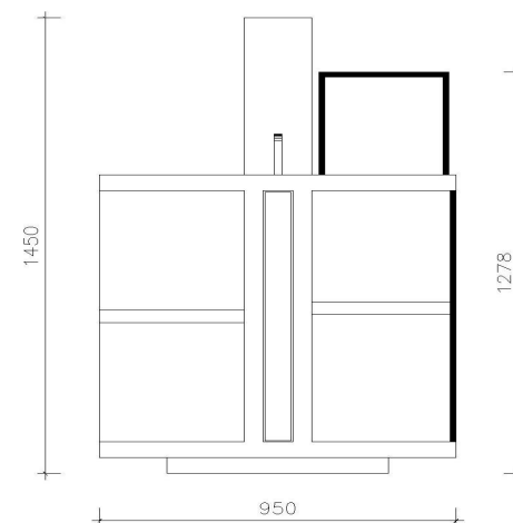
③ 右侧立面 SCALE 1/20
