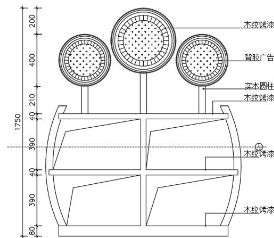
③ 立面图 SCALE 1/20
