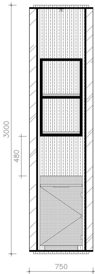
立面图 SCALE 1/30
