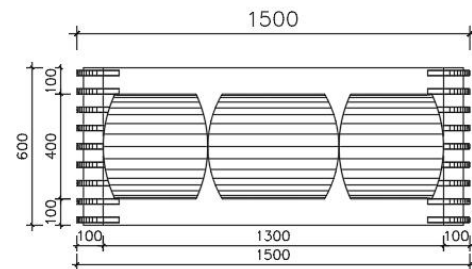
① 顶面图 SCALE 1/20
