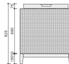
侧面图 SCALE 1/20
