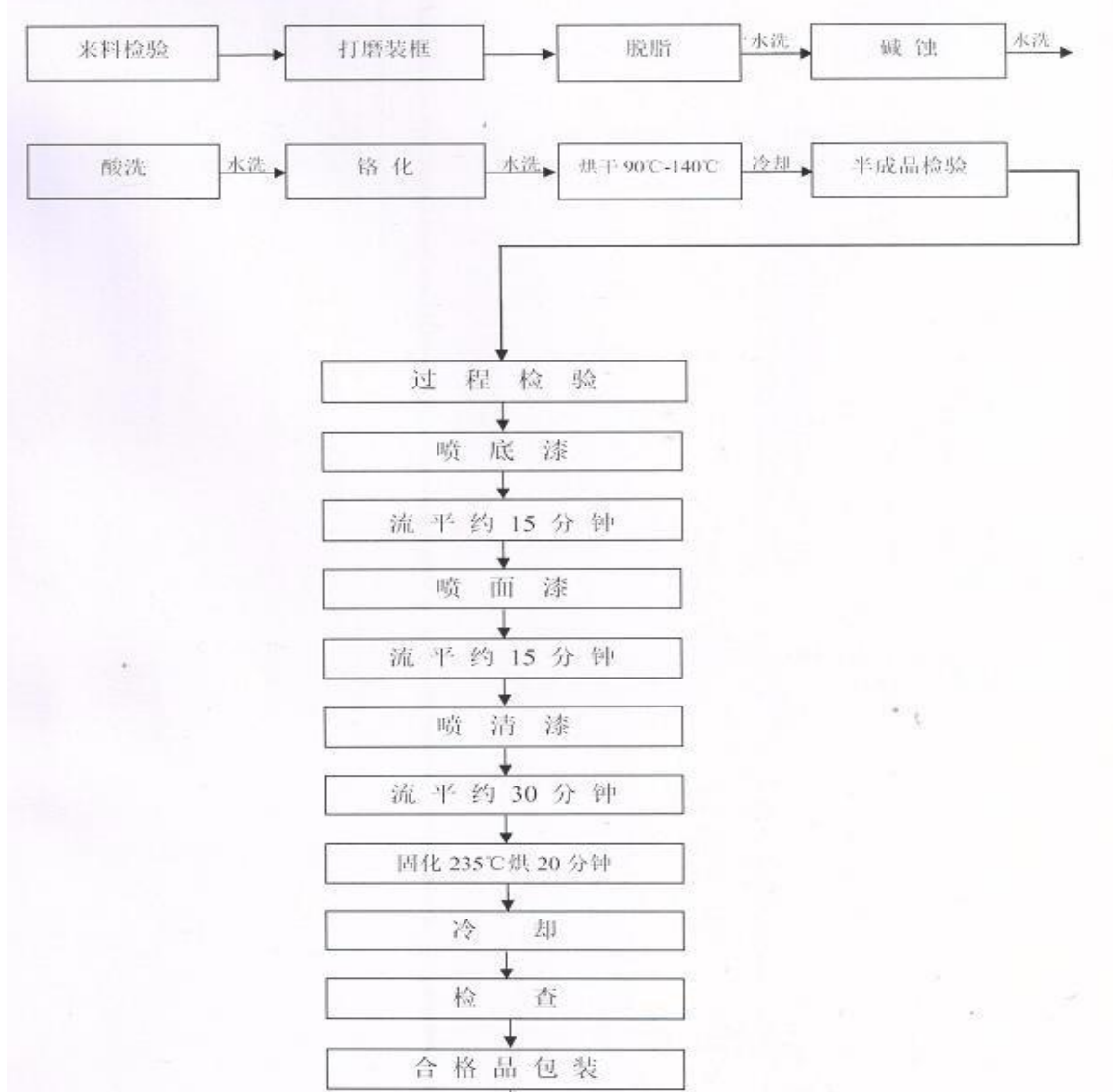
氟碳三涂生产流程图
