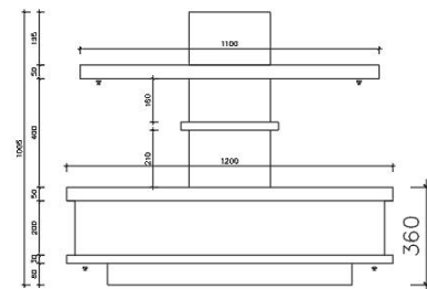
立面图 SCALE 1/20
