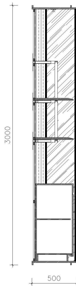
剖面图 SCALE 1/30
