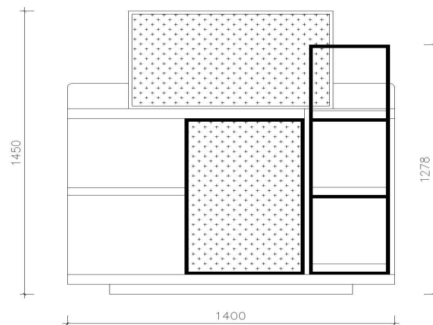
② 正立面 SCALE 1/20
