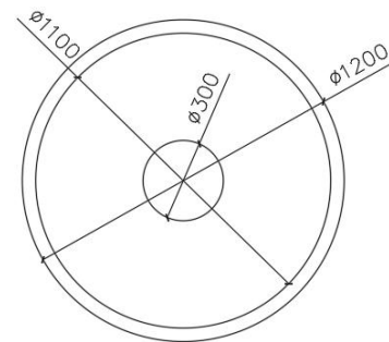
顶面图 SCALE 1/20
