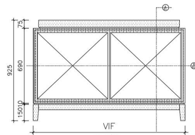
正面图 SCALE 1/20
